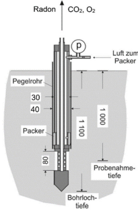
Abb. 1: Packer-Bodengassonde
